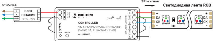
Рис. 2. Схема подключения контроллера SMART-SPI для управления светодиодной лентой SPI
