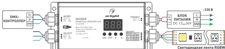
Рисунок 1. Подключение декодера SMART-K61-DMX-WP-SUF
