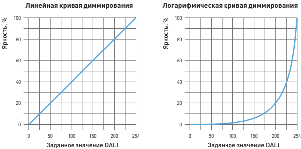
Рис. 4. Кривые диммирования
