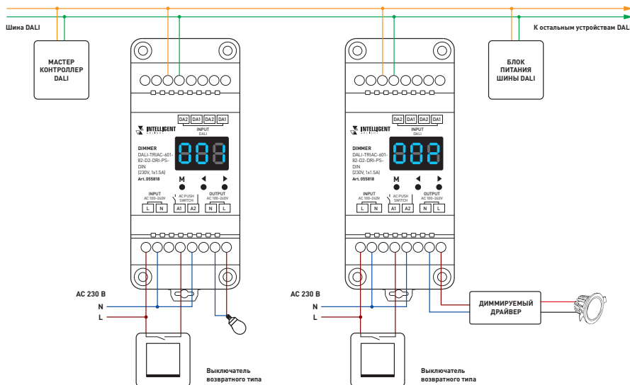
Рис. 2. Схема подключения диммера
