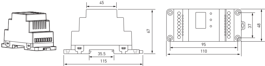
Рис. 1. Габаритный чертеж
